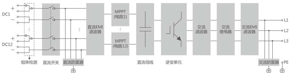
电路框图
