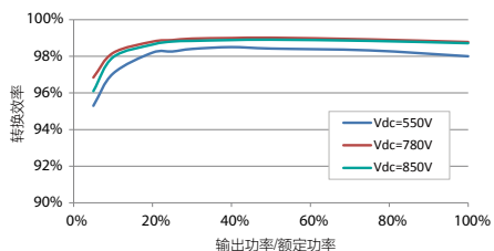
效率曲线
