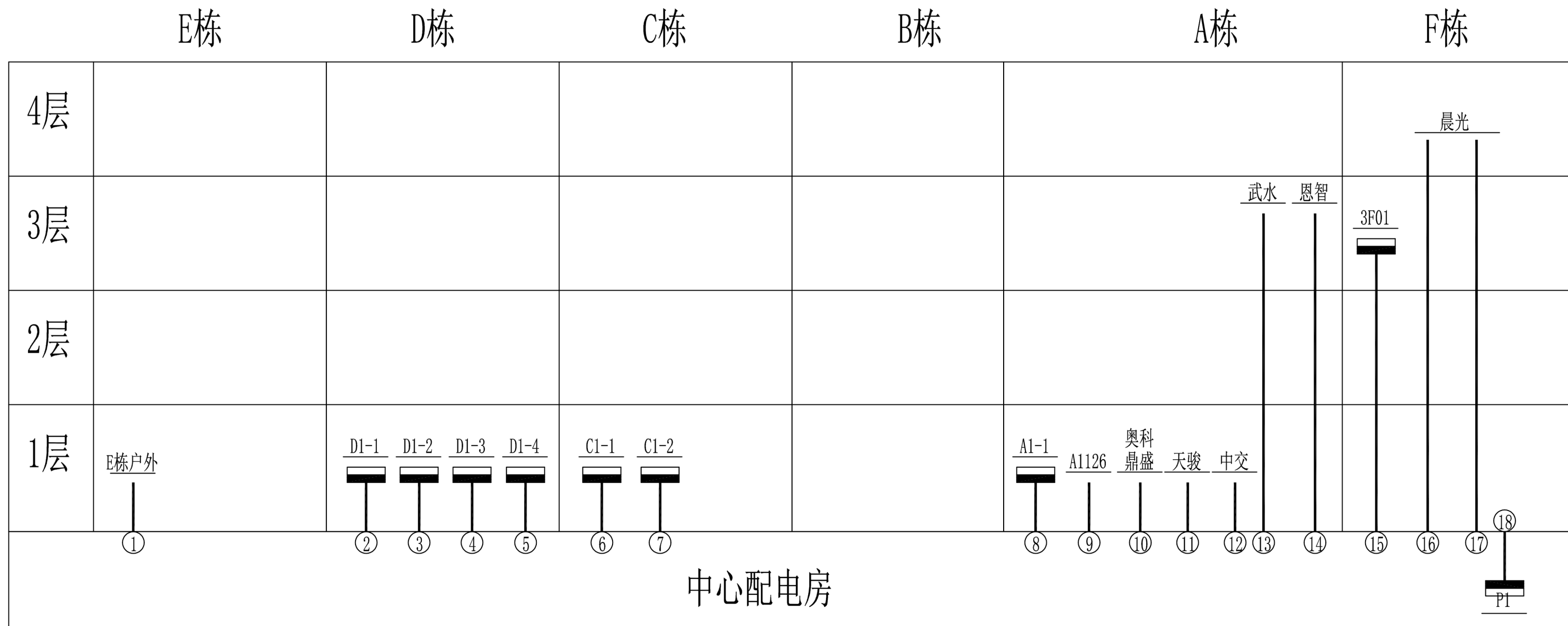
中心配电房 低压配电干线系统图
